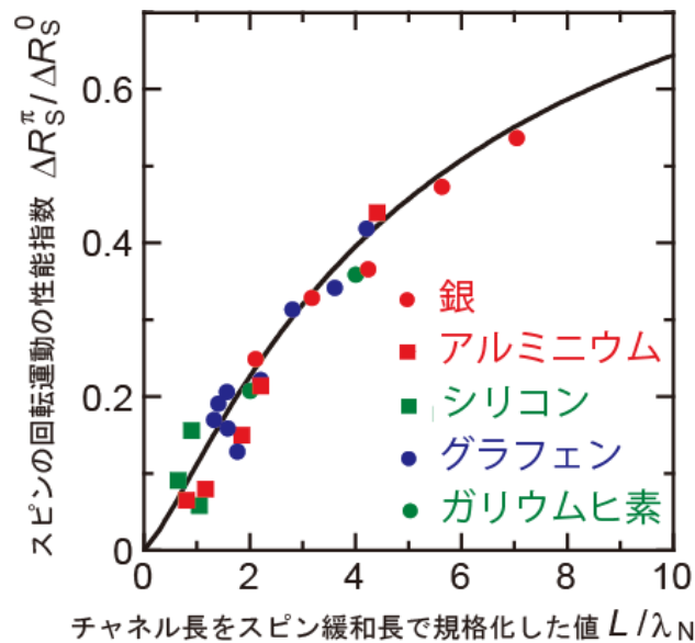
図 4 スピンの回転運動の性能指数の拡散距離依存性
